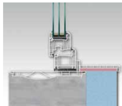
Verbessert den Wärmeschutz und spart Baukosten, denn Verputzarbeiten und Malerarbeiten entfallen. Abbildung bei Dämmung 10 cm.
