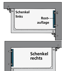
Aussparungen am Lichtschacht gemäß Kundenzeichnungen.
